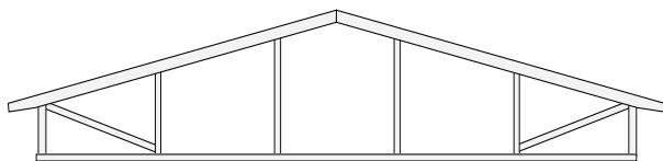
Spærfag med trempel og stol
