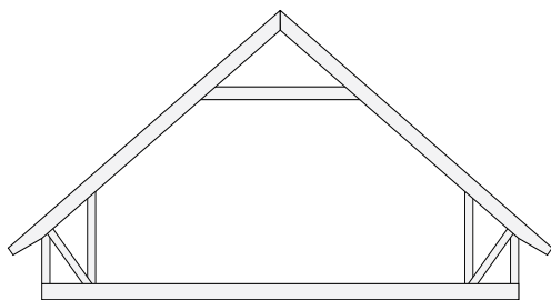
Hanebåndsspærfag
