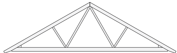
Fackverk
